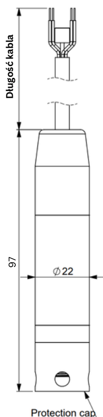
Sonda z osłoną ochronną z tworzywa sztucznego
