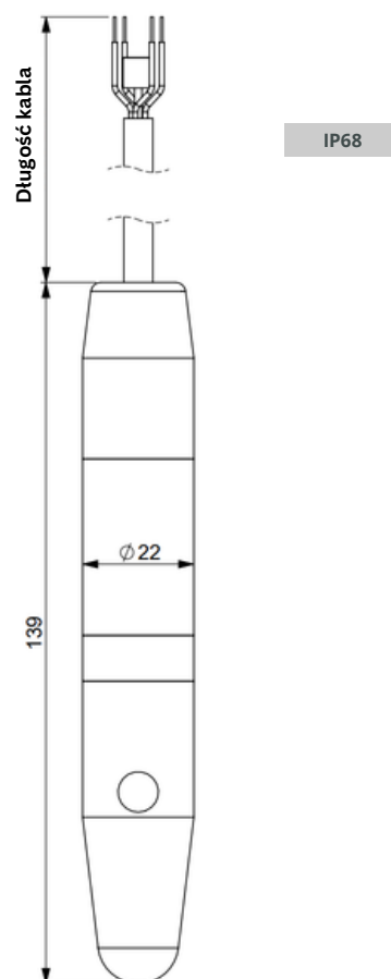
Sonda z obciążnikiem stalowym lub z tworzywa
